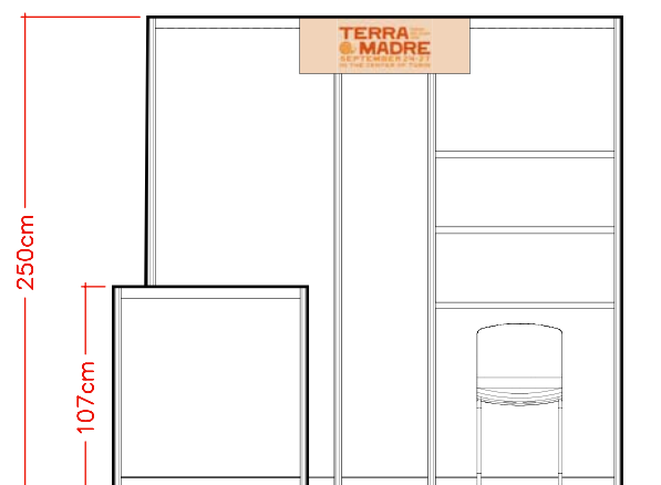
PROSPETTO / FRONT ELEVATION
